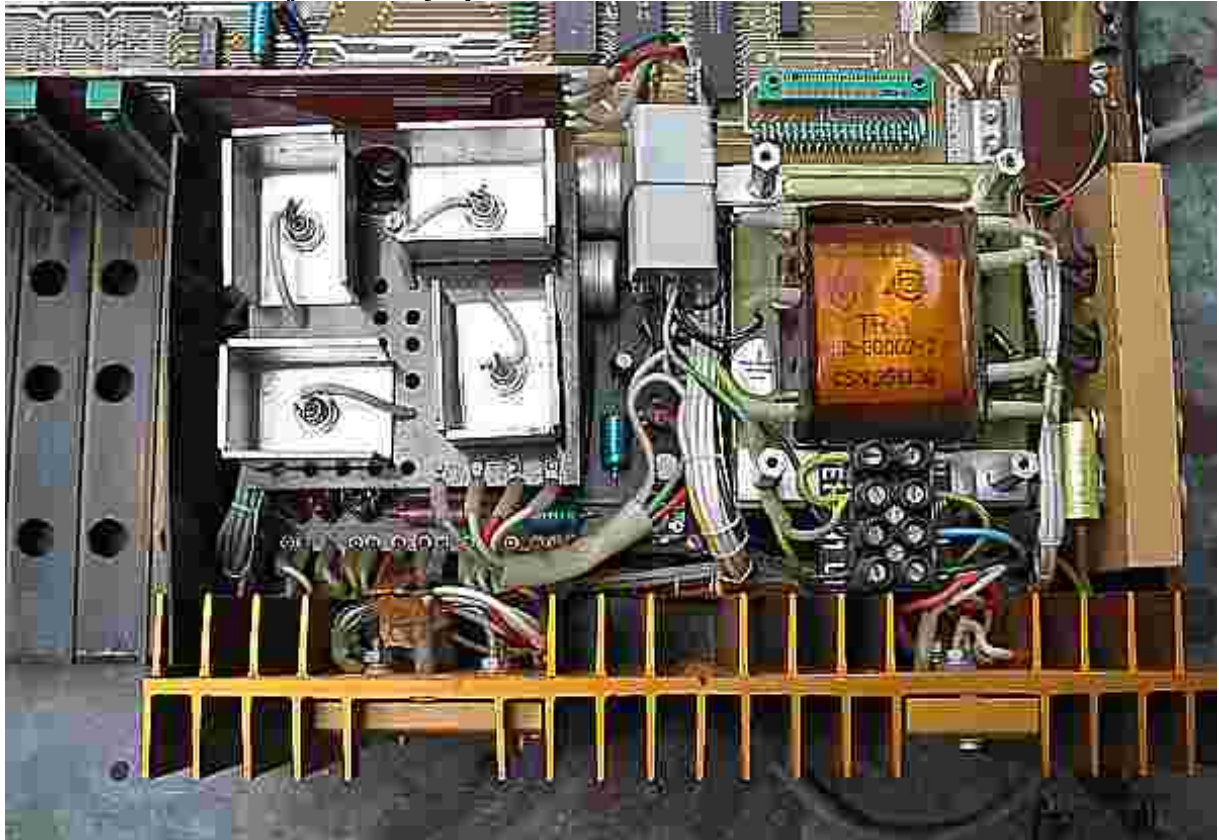
Zdroj IQ 151 vylepšené konstrukce s chladiči na diodách.
