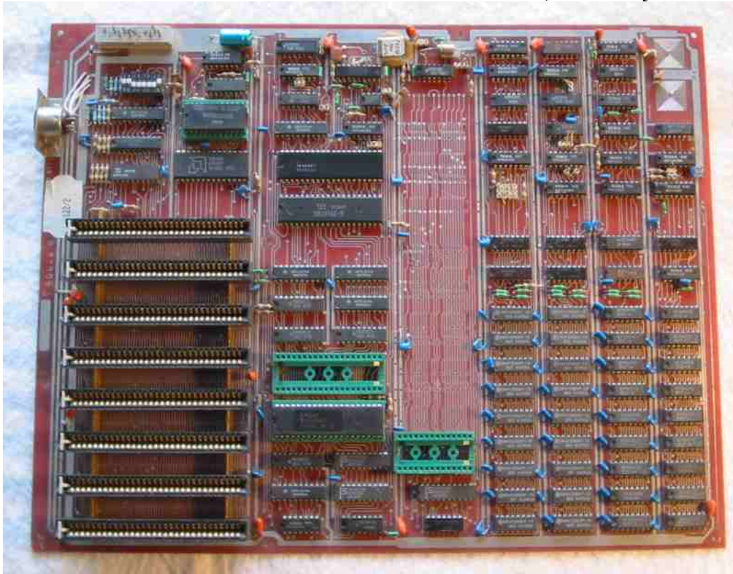
Základní deska – Mainboard PC XT se 640 Kb RAM, ZPA Nový Bor
